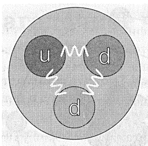
Рис. 1.2. Кварковая структура нейтрона
