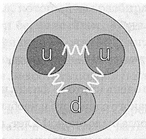
Рис. 1.3. Кварковая структура протона
