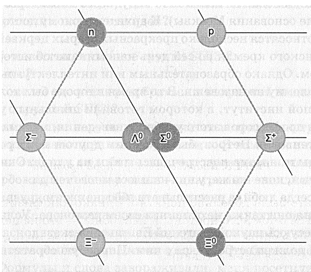
Рис. 1.4. Диаграмма октета
