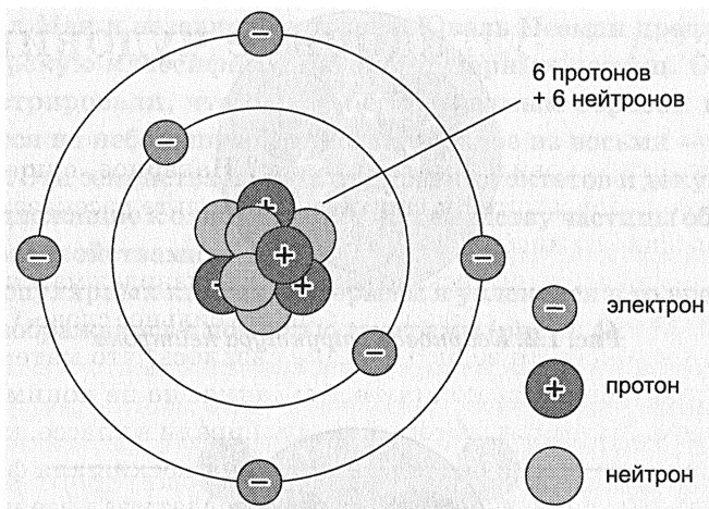
Рис. 1.1. Атом углерода
