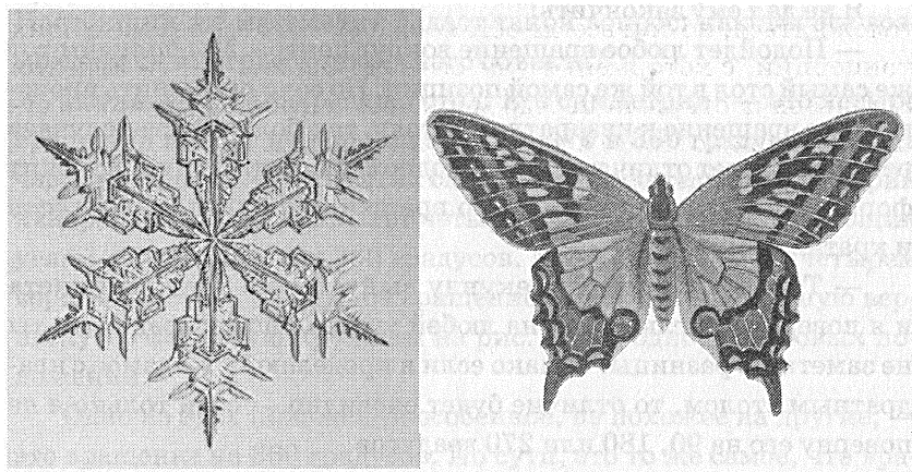
Рис. 2.1. Симметричные объекты
